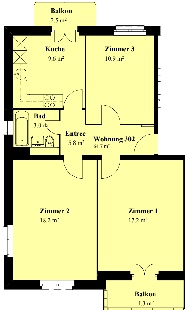
Grundriss 1:100
