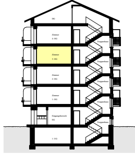
Schnitt 1:500
