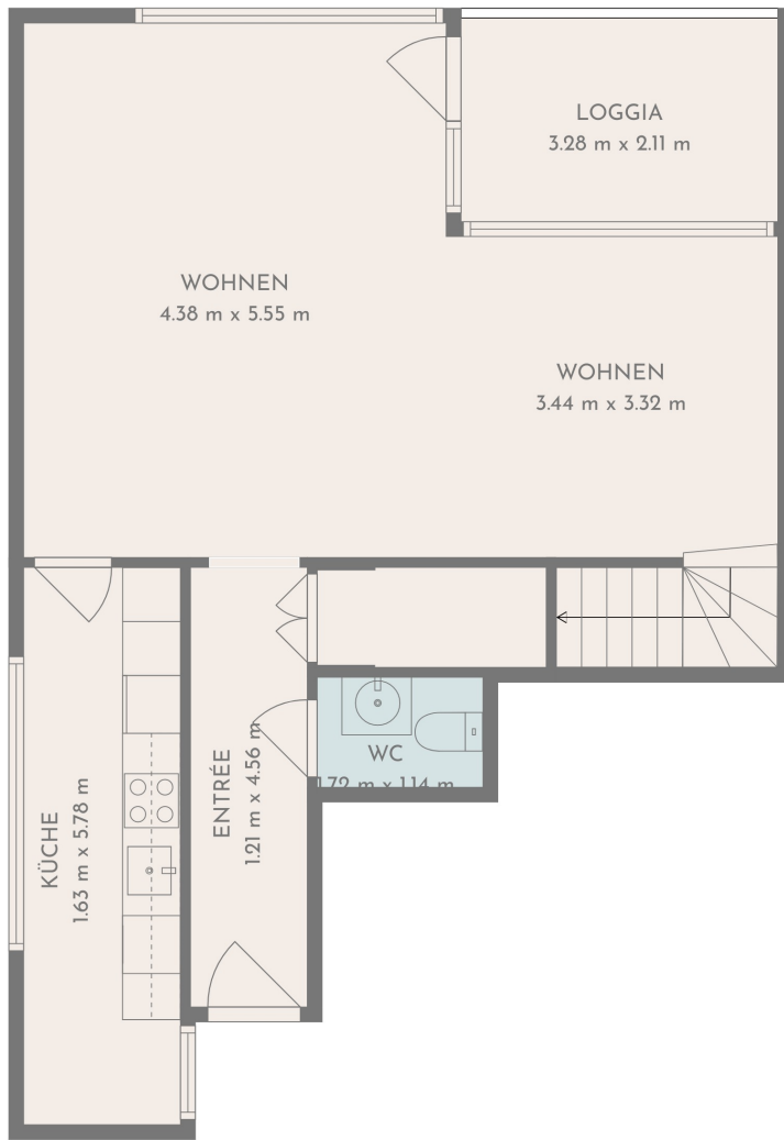
FUSSBODEN 1
