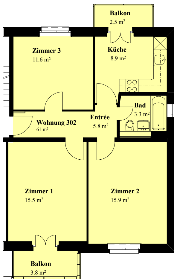
Grundriss 1:100
