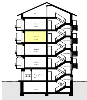
Schnitt 1:500
