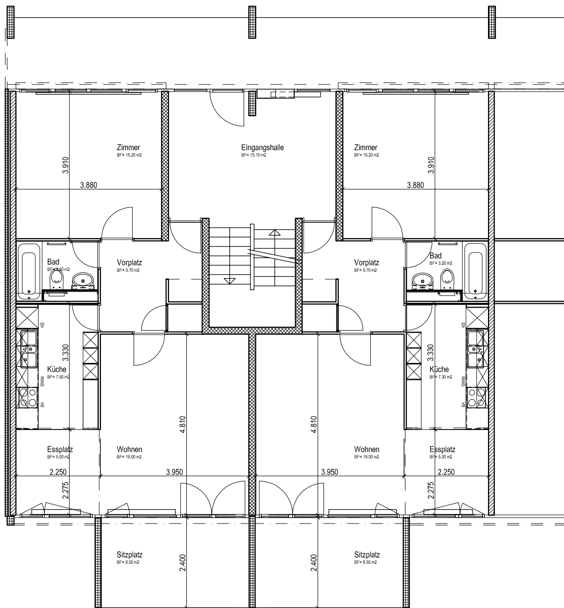
Grundriss 1:100
