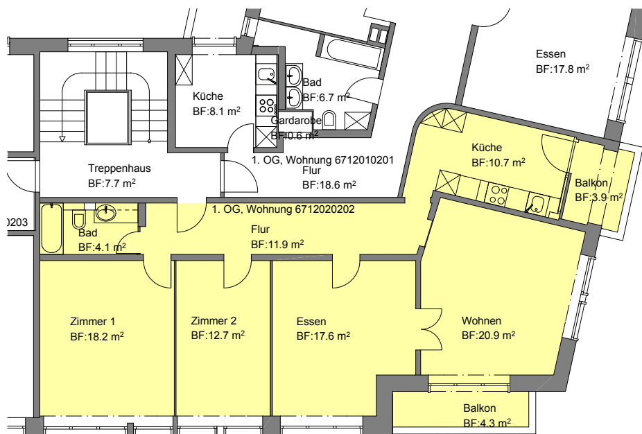
Grundriss 1:150
