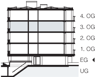
Schnitt
