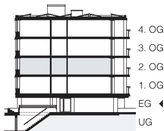
Schnitt
