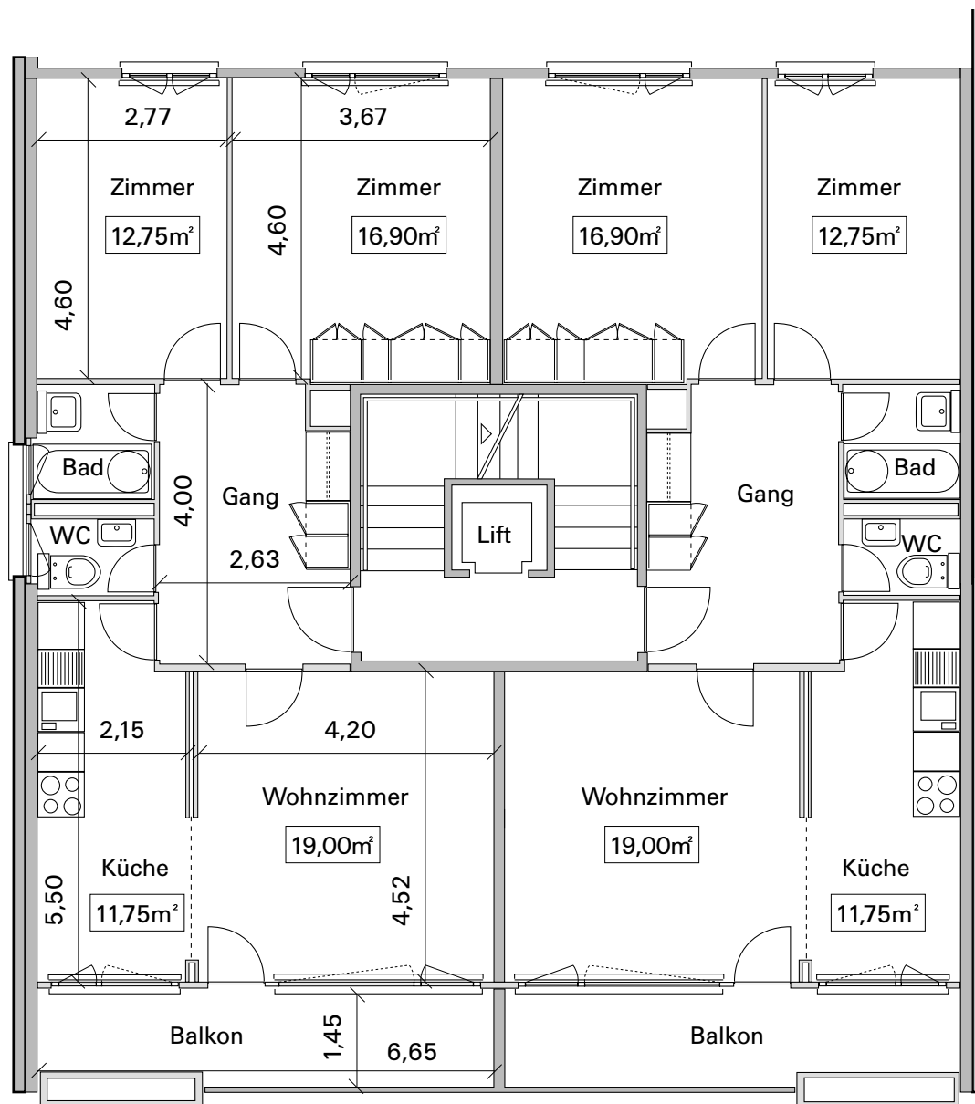
Grundriss 1:100
