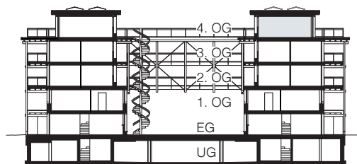
Schnitt
